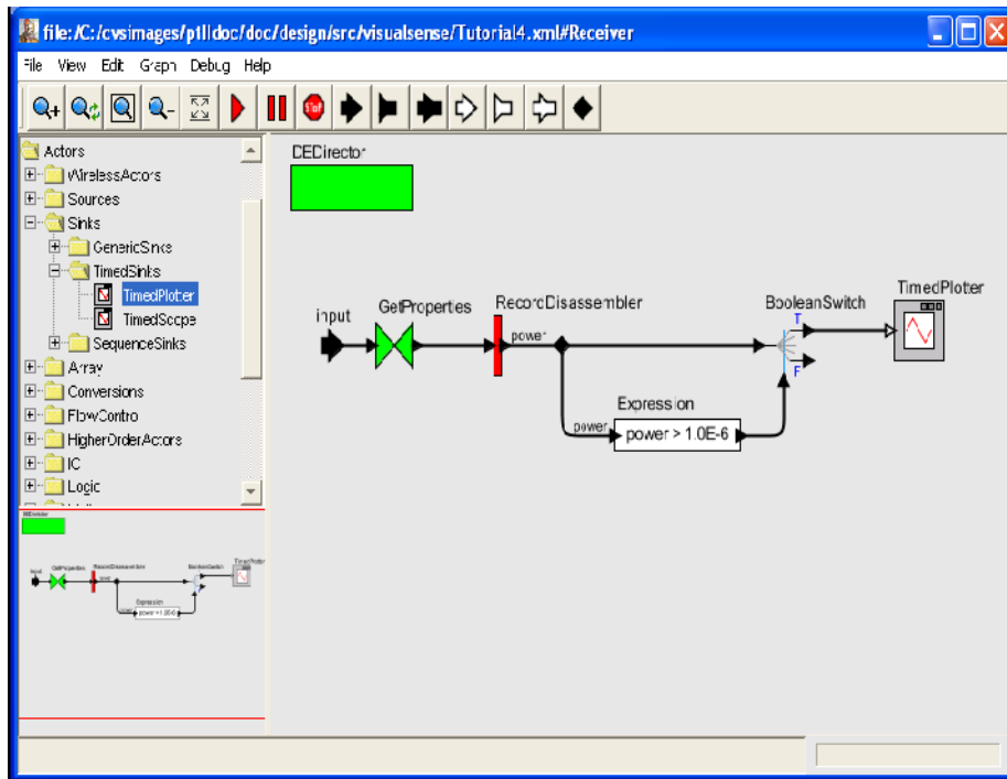
شکل (39) گیرنده توان دریافت شده را به صورت تابعی از زمان رسم می کند.
