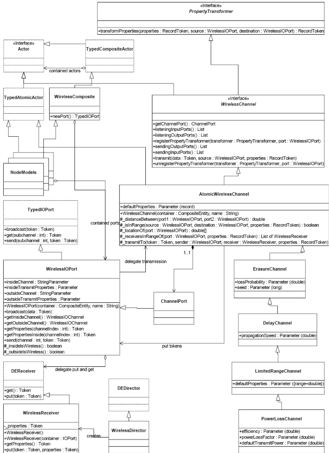
شکل (51) دیاگرام UML نشان دهنده کلاس های کلیدی برای مدل سازی شبکه حسگر بی سیم
